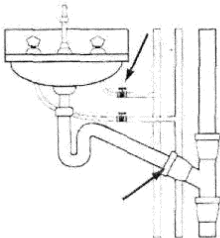
Раковина
